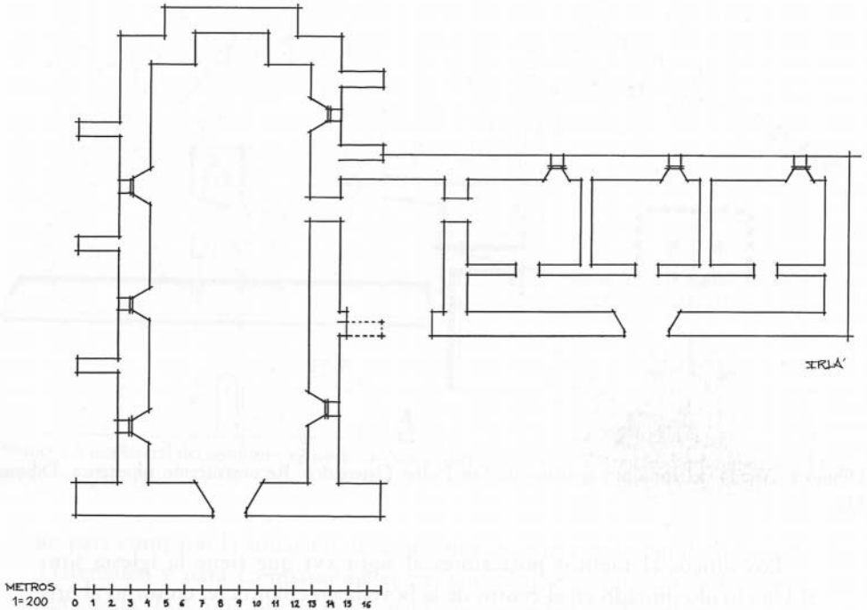
Dibujo 1. Planta del conjunto agustino de San Pedro Tlatemalco. Reconstrucción hipotética. Dibujo: Irla Granillo.
